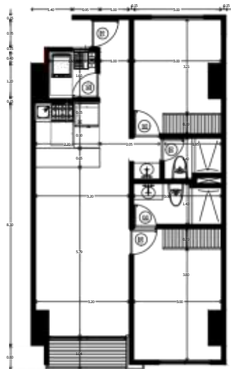
PLANTA
