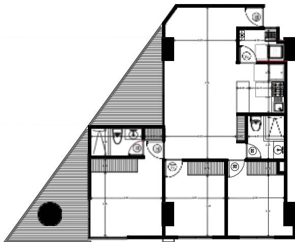
DEPARTAMENTO Tipo 05 (del PB-05 al 705)
